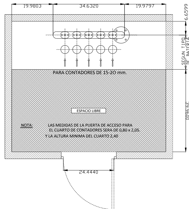
DIMENSIONES MINIMAS PARA CUARTO DE CONTADORES
