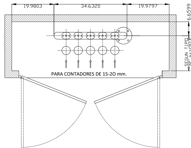
DIMENSIONES MINIMAS PARA ARMARIO DE CONTADORES
